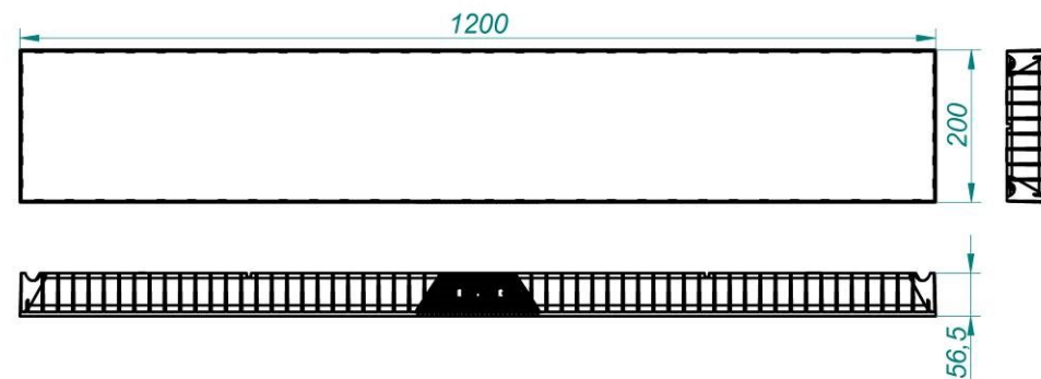
Рисунок 16 Светильник L-school 32
